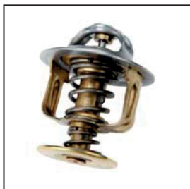
Termostato 83° Codigo: 3928639 Cummins 8.3L
