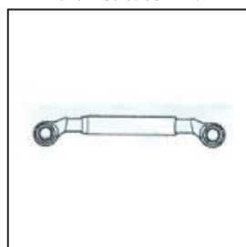
Barra Central Codigo: 488834 Scania K-124 Largo: 538mm.
