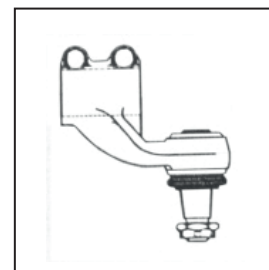
Terminal de Dirección Codigo: V6889484 Extremo direc. curvo der. Volvo B7 / B10 / B12 Largo: 168 mm.
