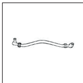
Barra de Dirección Codigo: V8195672 Barra dirección B10R Largo: 1099 mm.
