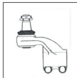
Terminal de Dirección Codigo: V6889483 Extre. direc. curvo izq. Volvo B7 / B10 / B12 Largo: 168 mm.
