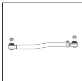
Barra de Dirección Código: A6344600005 Barra Dirección O500 Largo: 935 mm.
