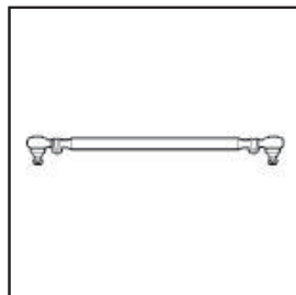
Barra Dirección Codigo: A6343300403 Largo: 1713 mm.
