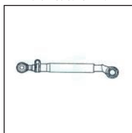
Barra Direc. Lateral Codigo: 1433532 Scania K-124 Largo: 635mm.
