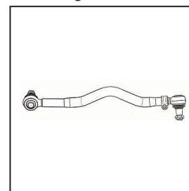
Barra de Dirección Codigo: V20745923 Largo: 1028 mm.
