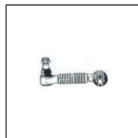
Bieleta Suspensión Código: A6343230316 Bieleta estab. del. der. O500 Largo: 375 mm
